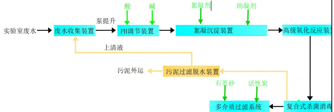
图 4-1 污水处理设备工艺图
