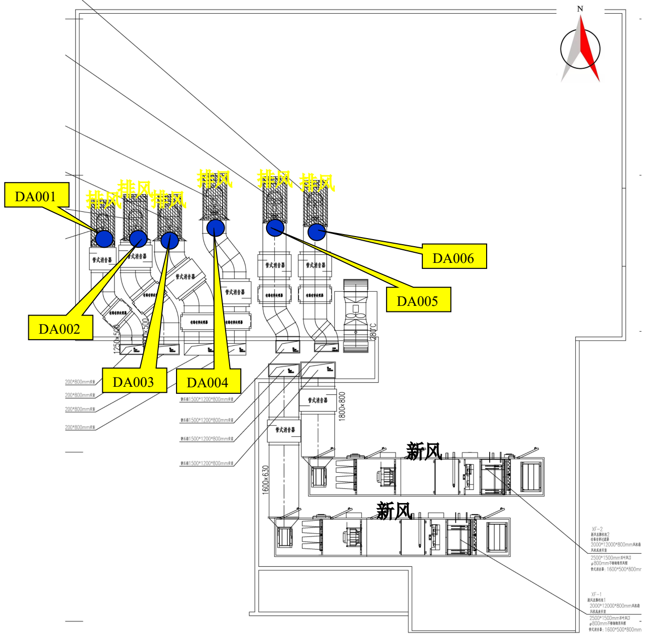
附图 4-7 项目实验室五层楼顶平面图
