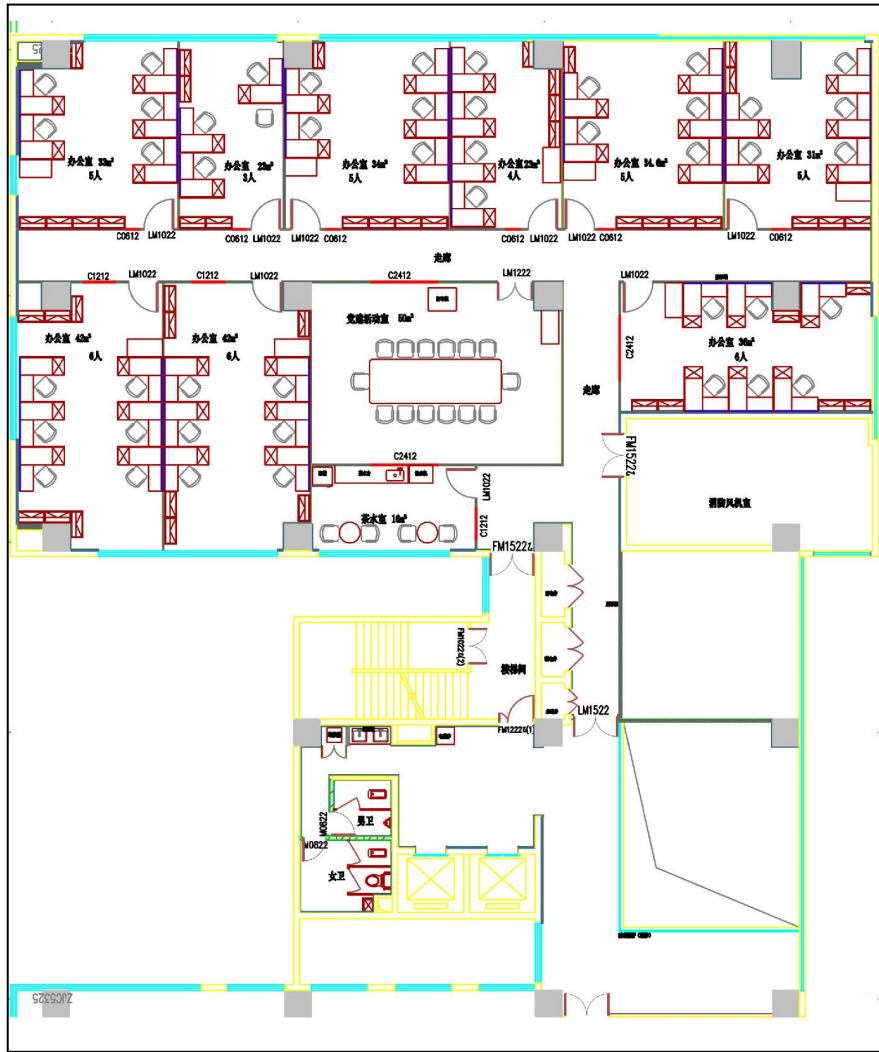
附图 4-3 项目实验室二层平面布置图
