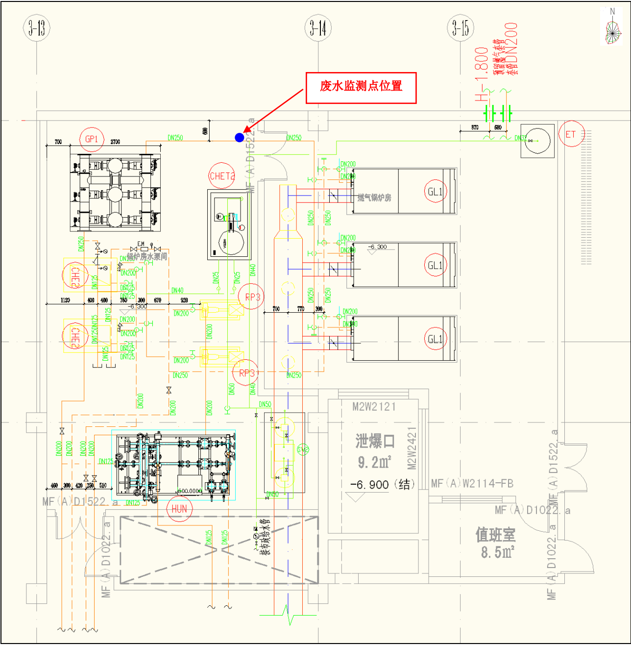
图 7-2 废水监测点位置示意图
