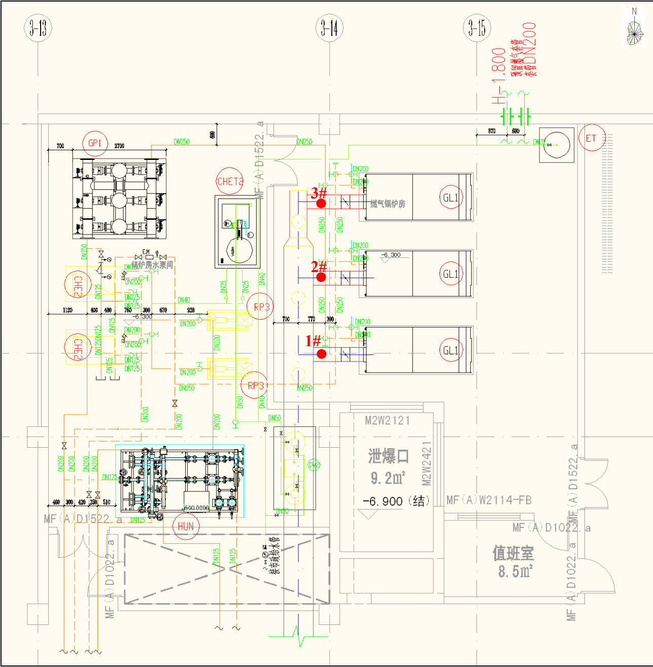
图 7-1 废气监测点位置示意图（● 废气监测点）
