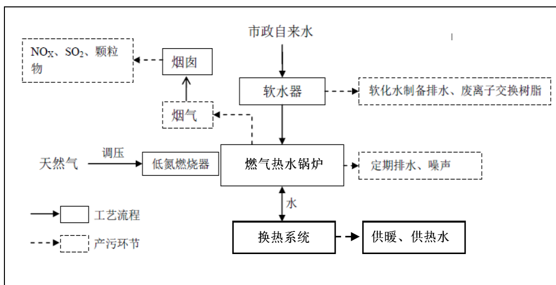
图 3-7 本项目工艺流程及产污环节图
